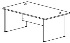
STANDARD TABLE iEXT 188 1800W x 800D x 750H iEXT 187 1800W x 700D x 750H iEXT 157 1500W x 700D x 750H iEXT 127 1200W x 700D x 750H
