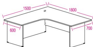
SUPERIOR COMPACT TABLE (L) iEXL 552 1500W x 1500W x 600D x 600D x 750H iEXL 1515 1500W x 1500W x 700D x 600D x 750H iEXL 1815 1800W x 1500W x 700D x 600D x 750H
