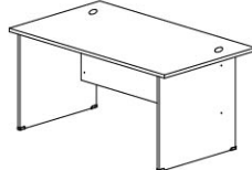
STANDARD TABLE IGT 188 1800W x 800D x 750H IGT 187 1800W x 700D x 750H IGT 157 1500W x 700D x 750H IGT 127 1200W x 700D x 750H
