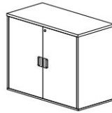
SWINGING DOOR CABINET IGD 880 800W x 400D x 820H
